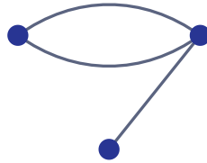
Multigraph
